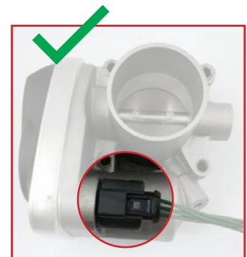
Die Steckerbuchse muss fest an der Drosselklappe einrasten.
